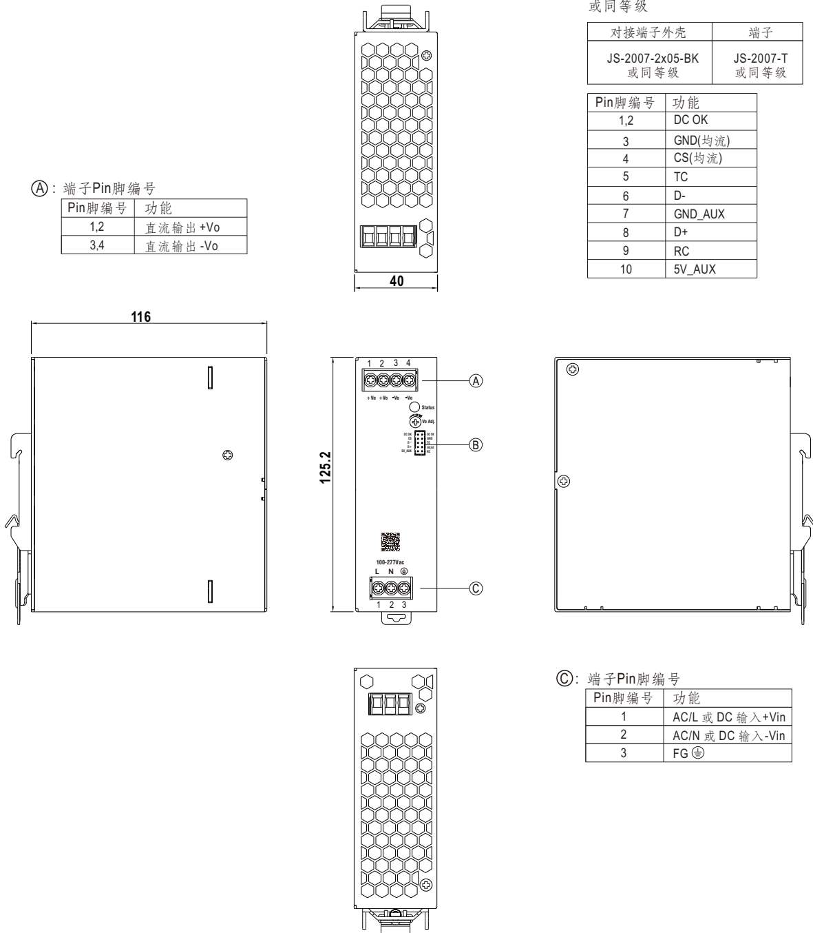
Ⓑ: 控制端子Pin脚编号 :JS-2008R-2x05 或同等级
