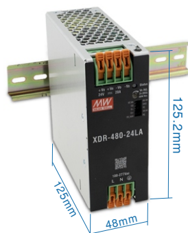
(XDR-480-xxLA)
